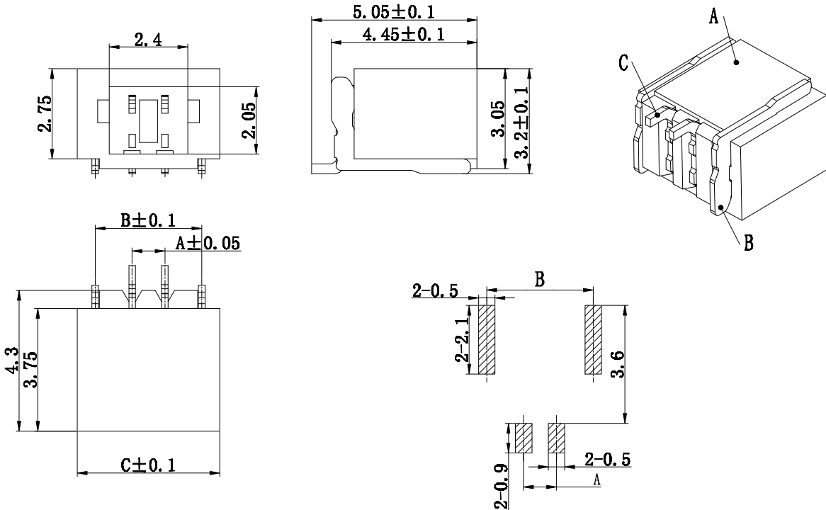
PCB参考图
