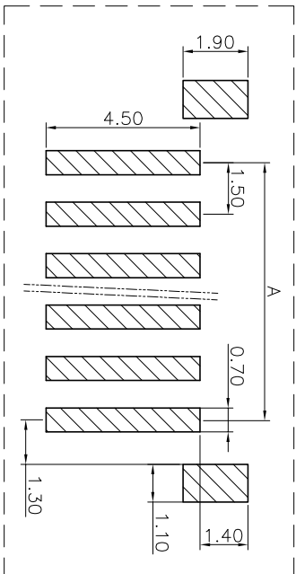
PCB LAYOUT TOL.: ±0.05
