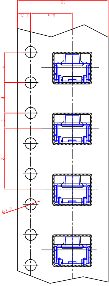
载带尺寸图
