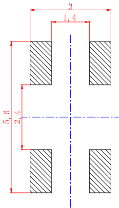
P C B 参考图
