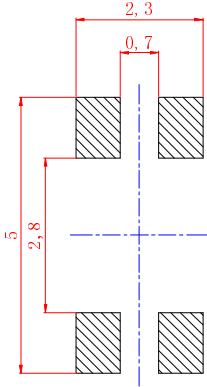
P C B 参考图
