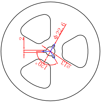
编带盘尺寸图
