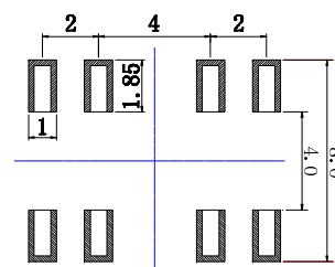
PCB参考图
