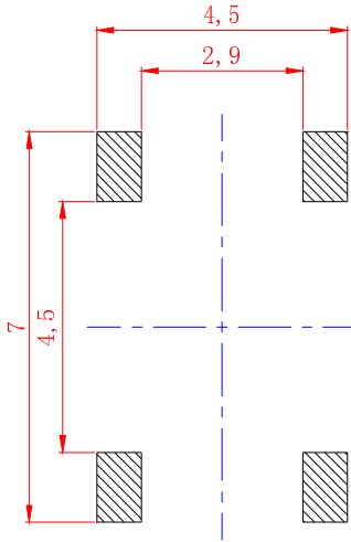
P C B 参考图
