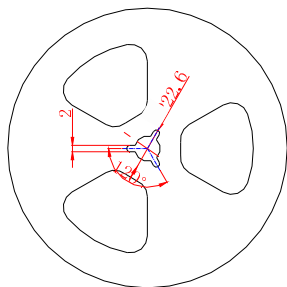
图 带盘尺寸
