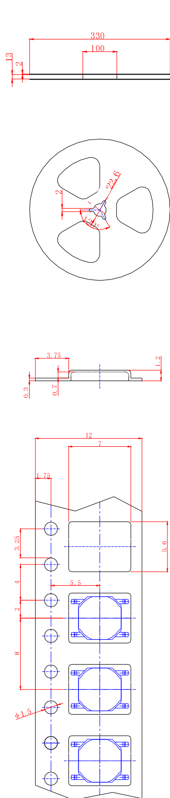
图 带盘尺寸
