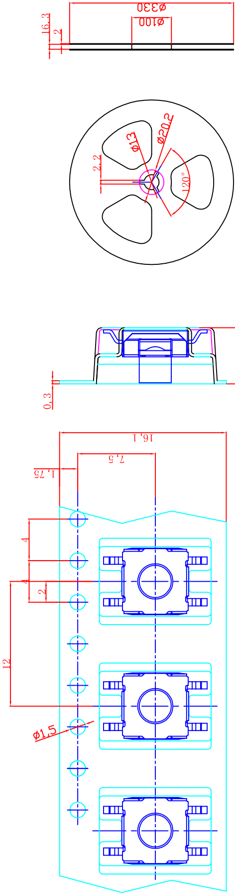
载带尺寸图
