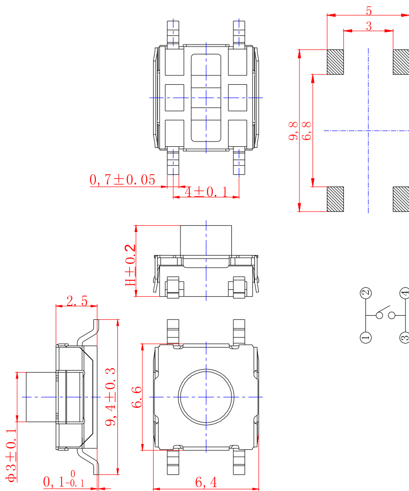
PCB 参考图
