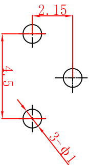
PCB参考图
