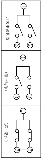
电器原理图
