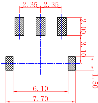
PCB参考图
