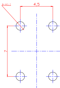
PCB 参考图
