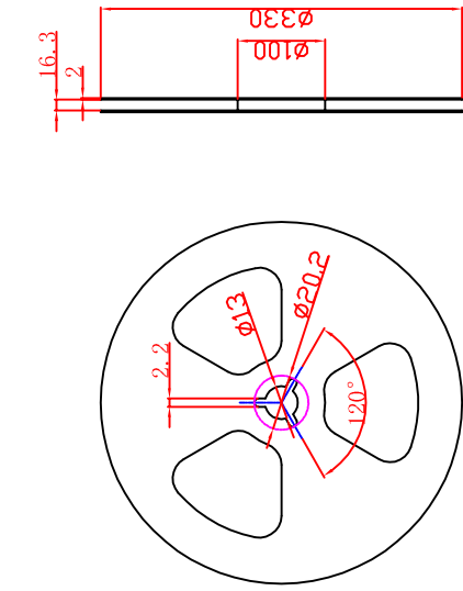
编带盘尺寸图
