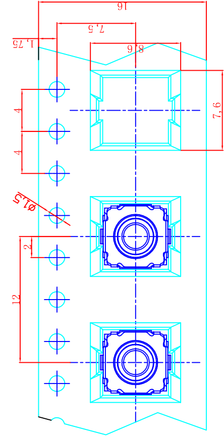
载带尺寸图
