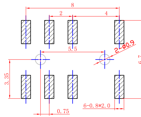
P C B 参考图
