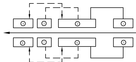
电器原理图
