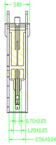
截面 B-B
