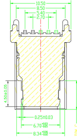
截面 A-A
