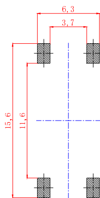
PCB. 焊接图
